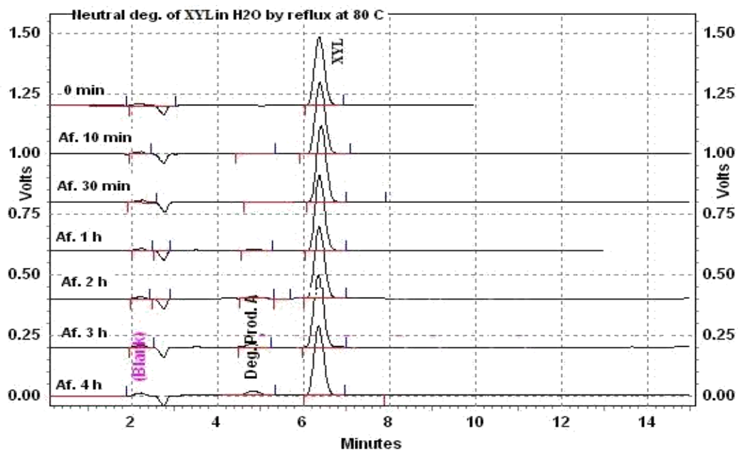
Fig. 5: Chromatograms of 100 ug/ml XYL in Neutral condition standard, 0 min, 10 min, 30 min, 60 min, 120 min, 180 min and 240 min (4hr) reflux at 80 o C
